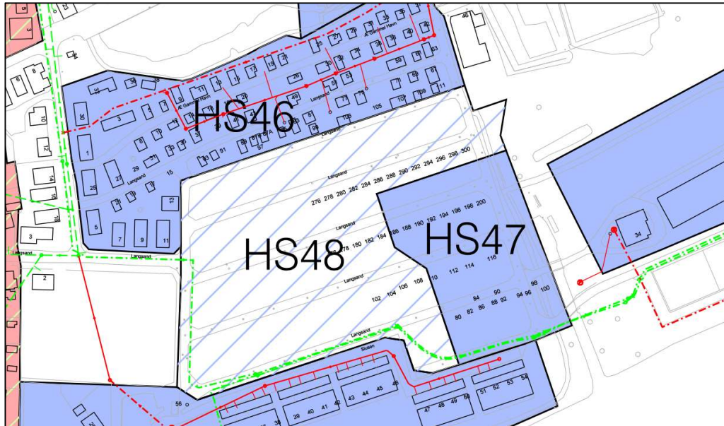
Figur 6 Udsnit af Hvide Sande med de berørte oplande HS47 og HS48. Ringkøbing-Skjern Forsyning A/S kloakerer oplandene for spildevand, mens grundejerne selv skal håndtere afledning af tag- og overfladevand.
