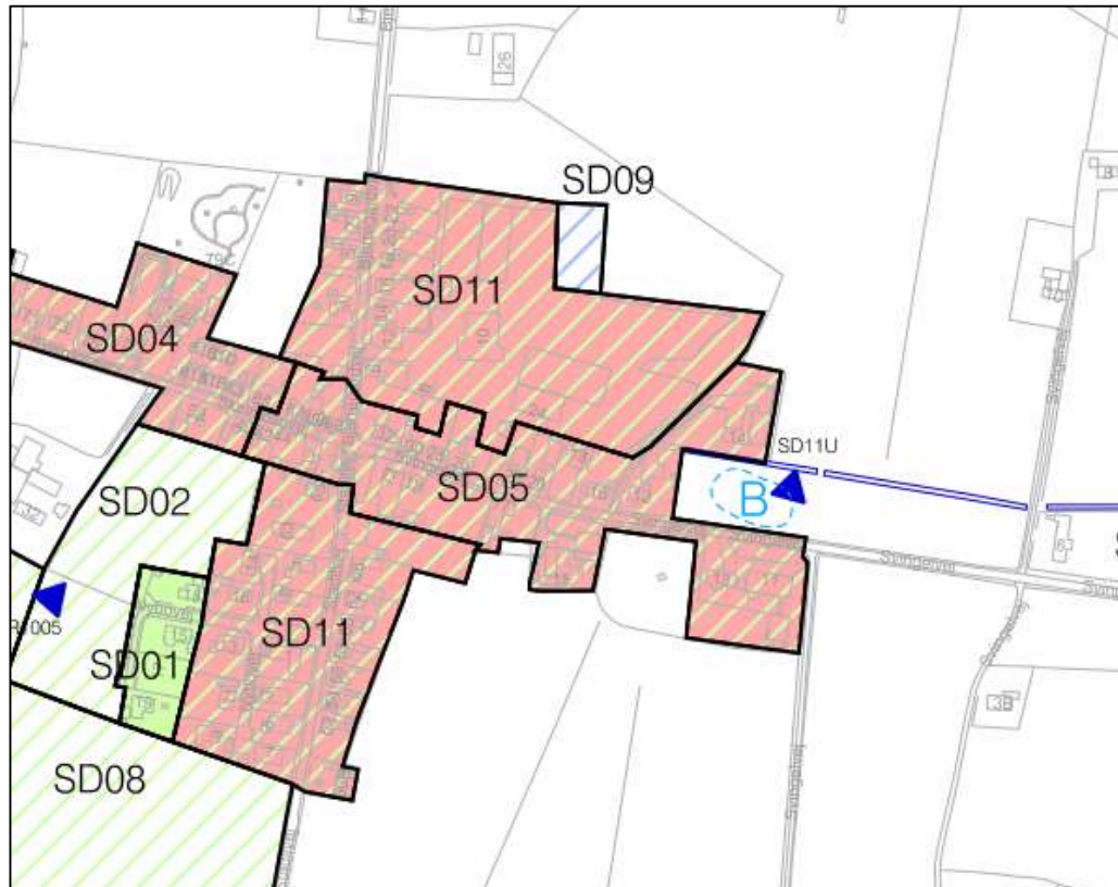
Figur 3 Separering af det fælleskloakerede opland SD11, så hele Stadil bliver separeret. Øvrige separeringer af fælleskloakken i Stadil er allerede besluttet gennem Spildevandsplan 2019-2027.
